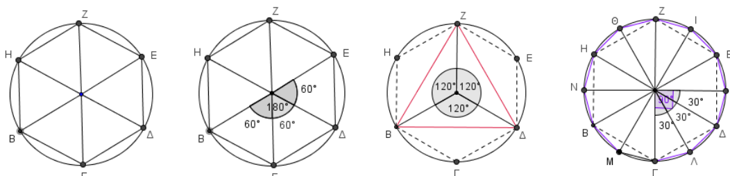
Σχήμα 1: Το εξάγωνο ως γεωμετρικό μοντέλο τριχοτόμησης γωνιών 180^\circ , 360^\circ και 90^\circ
