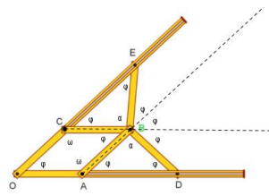
Σχήμα 6: Εξήγησης της λειτουργίας της συνδεσμολογίας του Ceva ως εργαλείο τριχοτόμησης γωνίας στο φύλλο εργασία (αριστερά) και σε ψηφιακό αντίγραφο (δεξιά)
