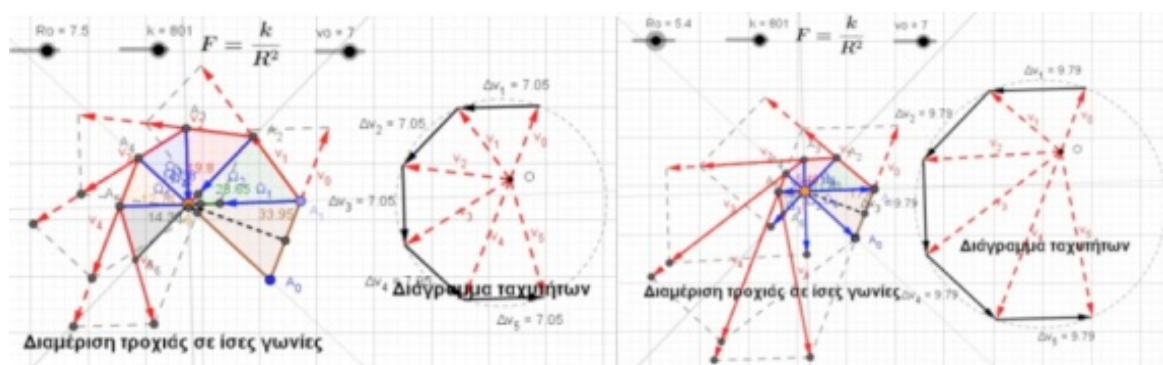
Εικόνα 6: Διάγραμμα ταχυτήτων για διαφορετικές αρχικές αποστάσεις από τον Ήλιο
