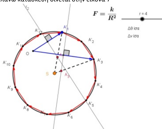
Εικόνα 7: Στο κέντρο του κύκλου τοποθετούμε τον Ήλιο. Το κέντρο των ταχυτήτων O είναι αυθαίρετο. Έστω OA_1 η ταχύτητα του πλανήτη στη θέση 1. Το σημείο τομής της μεσοκαθέτου OA_1 και της SA_1 είναι η θέση του πλανήτη
