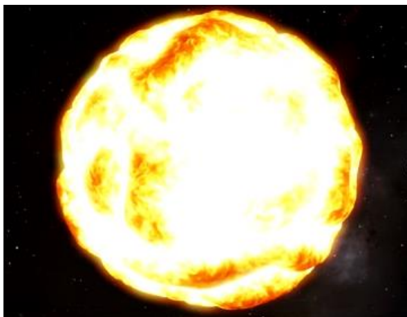
Εικόνα 13: Κόκκινος Υπεργίγαντας
