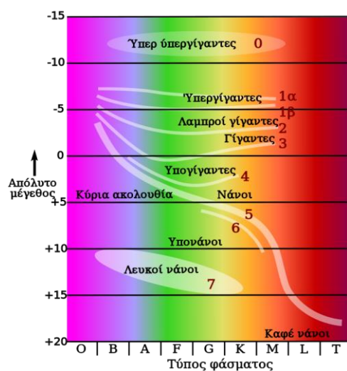
Εικόνα 2: Διάγραμμα Χέρτζσπρουγκ-Ράσελ
