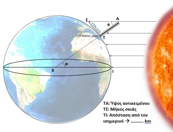
Σχήμα 2: Προσδιορισμός επίκεντρης γωνίας φ και τόξου Γης, μέσω της μέτρησης του ύψους του αντικειμένου και του μήκους της σκιάς κατά την εαρινή ισημερία.
