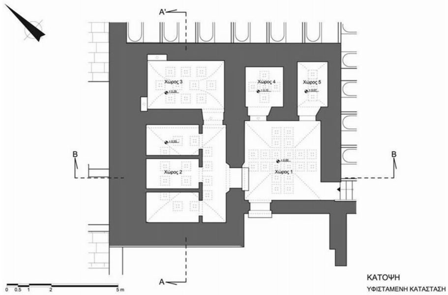
ΕΙΚΟΝΑ 15: Η κάτοψη του χαμάμ
