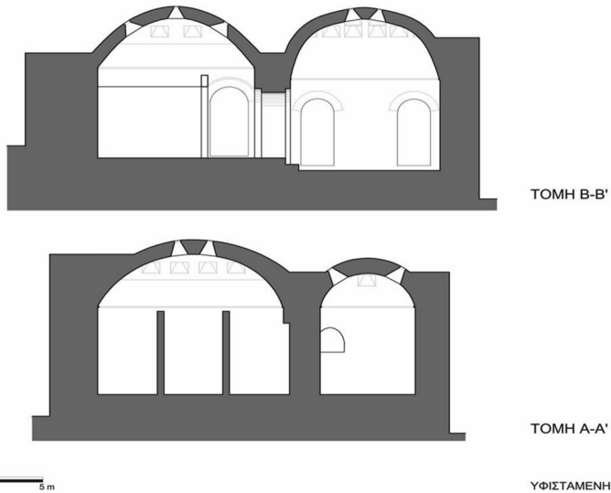
ΕΙΚΟΝΑ 27: Σχεδιαστικές τομές του χαμάμ. Υφιστάμενη κατάσταση
