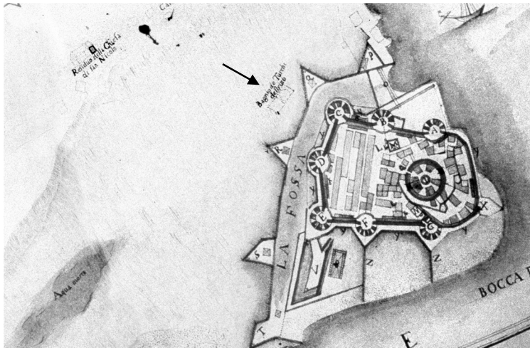
ΕΙΚΟΝΑ 3: Αποτύπωση του κάστρου της Μπούκας και του χαμάμ (βέλος). Λεπτομέρεια χειρόγραφου σχεδίου του G.L. Mauro του 1685 (ΚΑΡΑΜΠΕΛΑΣ 2010, 428, εικ. 10)
