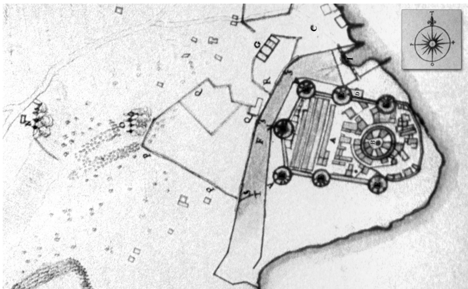
ΕΙΚΟΝΑ 2: Αποτύπωση του κάστρου της Μπούκας. Στη θέση G το χαμάμ. Λεπτομέρεια χειρόγραφου σχεδίου αγνώστου του 1684 (ΚΑΡΑΜΠΕΛΑΣ 2010, 428, εικ. 9)
