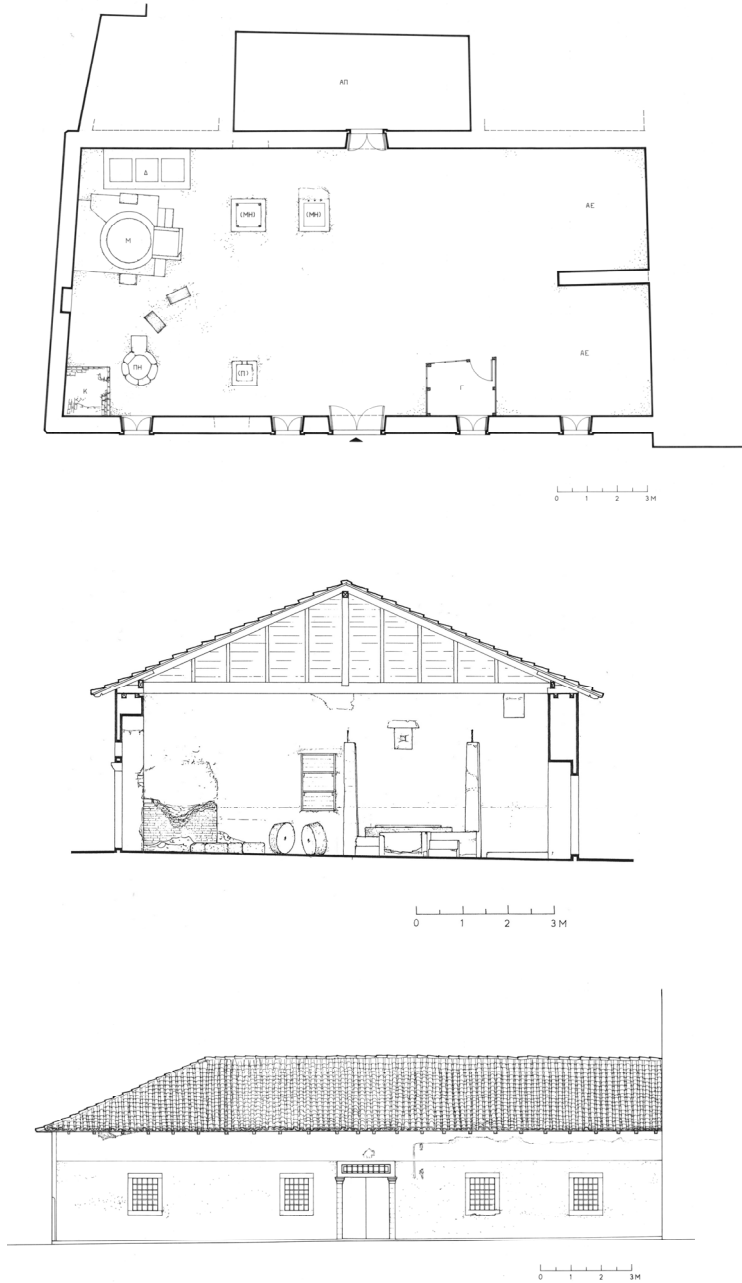
ΕΙΚΟΝΑ 8: Ελαιοτριβείο οδών Χαρ. Μούσκου 22 και Σάνδριτζ. Α. Κάτοψη, Β. Τομή ΑΑ, Γ. Δυτική Όψη
