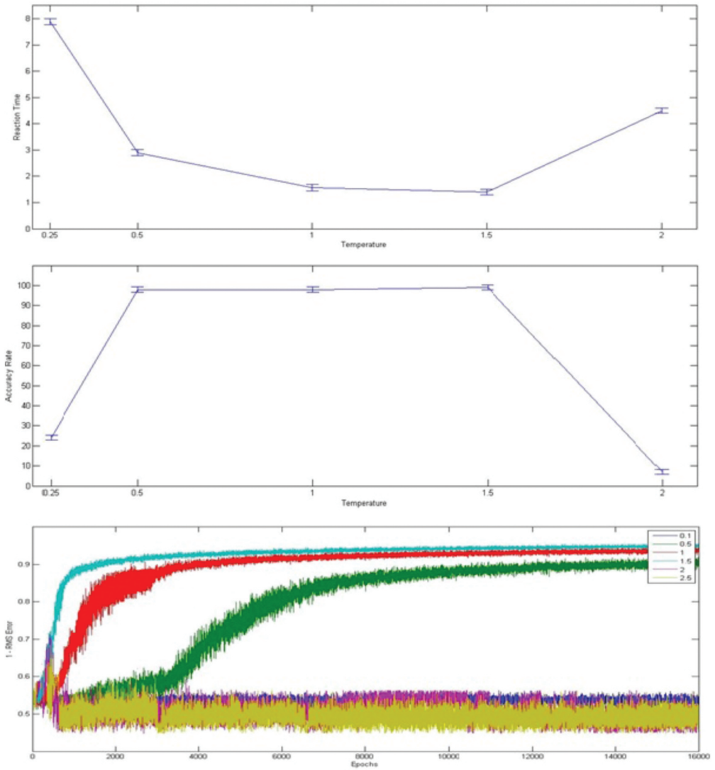
Σχήμα 2 Χρόνος αντίδρασης, ακρίβεια και σφάλμα RMS για τη σταθερά της συνάρτησης
