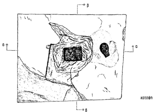
Γ. Βελένης, Εικ. 1. Έπιγραφή βάση από την αρχαία Άγορά της Θεσσαλονίκης. α) Κύρια όψη, β) τομή α - α, γ) τομή β - β, δ) κάτοψη
