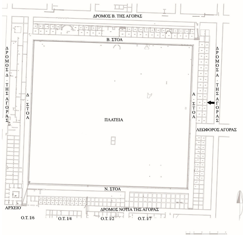
Εικ. 10. Κάτοψη της Αγοράς της Πέλλας. Σημειώνεται η θέση του χώρου 29. Αρχείο Πανεπιστημιακής Ανασκαφής Αγοράς Πέλλας, Α.Π.Θ.
