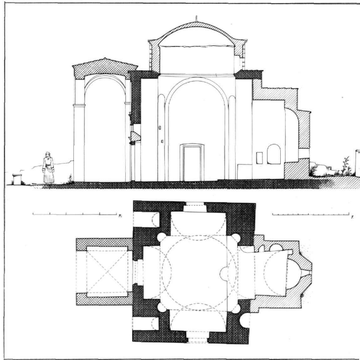
Εικ. 2. Μονή Ζωοδόχου Πηγής. Κάτοψη και τομή τής λιτής στην ύπάρχουσα κατάσταση.
