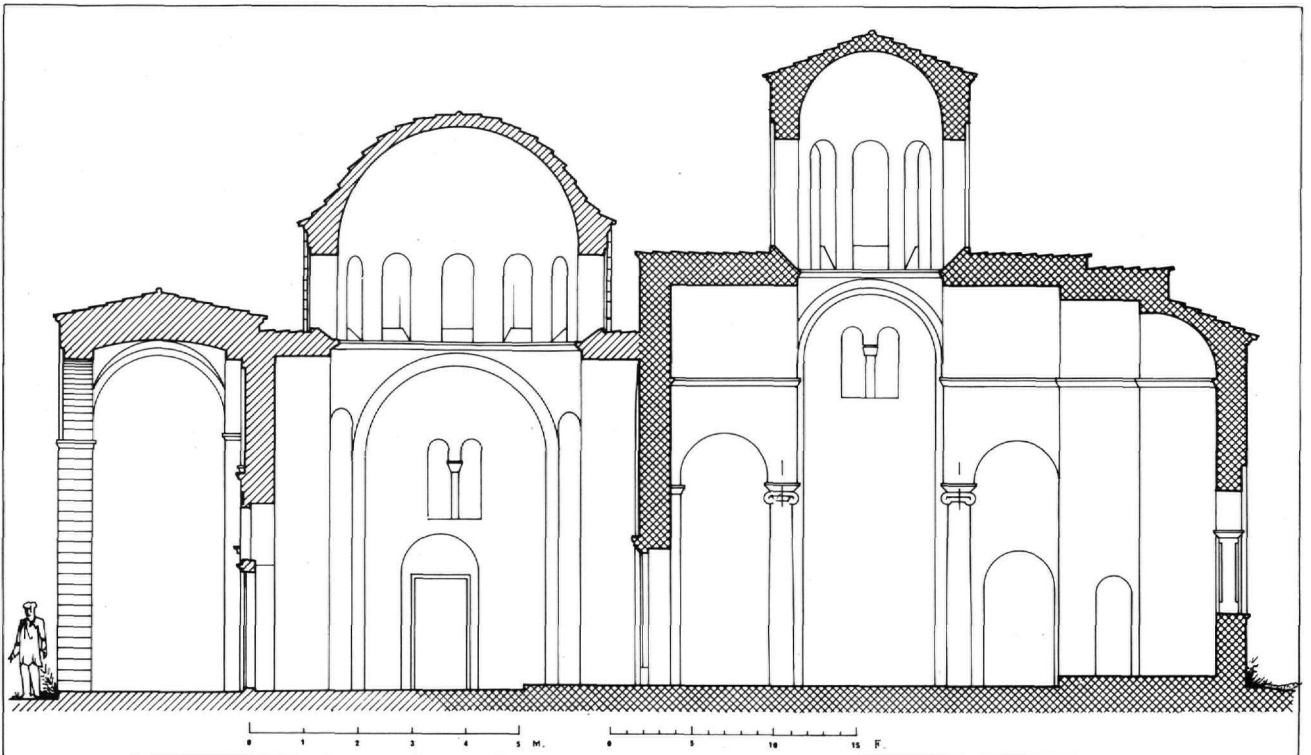
Εικ. 2. Μονή Ζωοδόχου Πηγής. Κάτοψη και τομή της λιτής στην υπάρχουσα κατάσταση.
