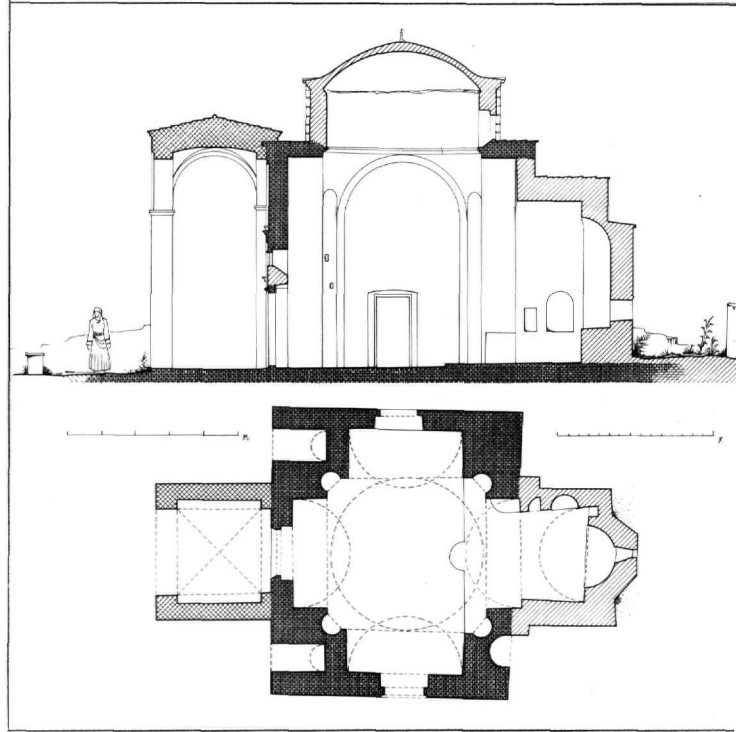
Εικ. 2. Μονή Ζωοδόχου Πηγής. Κάτοψη και τομή της λιτής στην υπάρχουσα κατάσταση.
