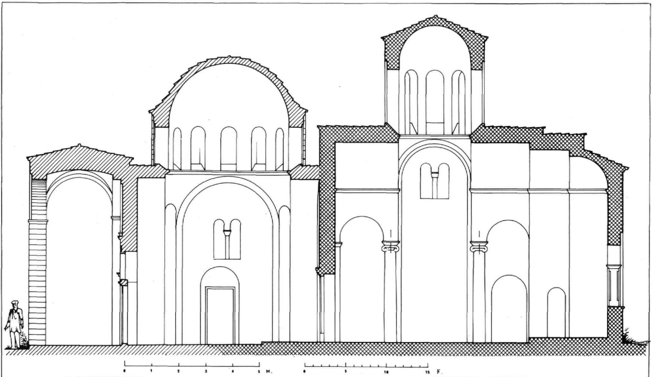
Εικ. 2. Μονή Ζωοδόχου Πηγής. Κάτοψη και τομή τής λιτής στην ύπάρχουσα κατάσταση.
